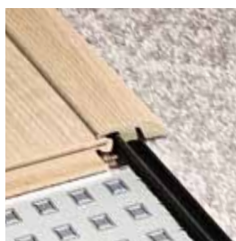
1. Profil łączący 1850 X 43,7 X 12,5 MM
